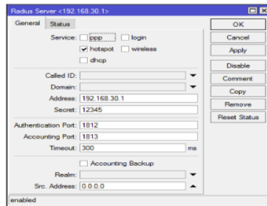
Gambar 18. Konfigurasi RADIUS
