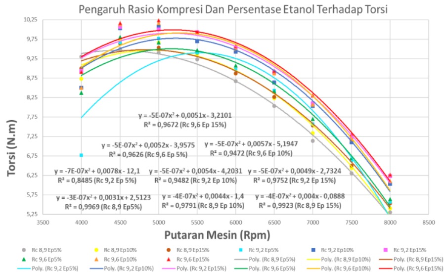
Gambar 3. Grafik Hasil Pengujian Torsi
