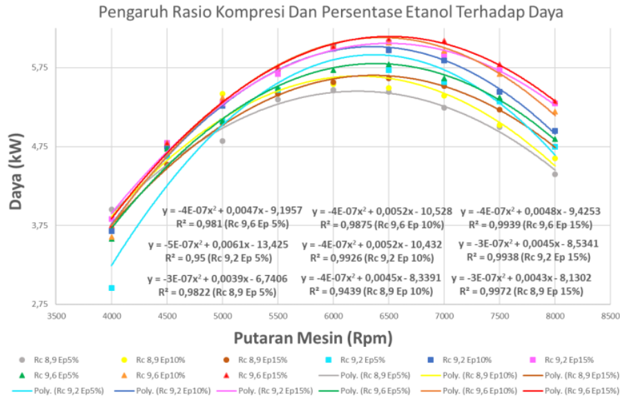
Gambar 2. Grafik Hasil Pengujian Daya
