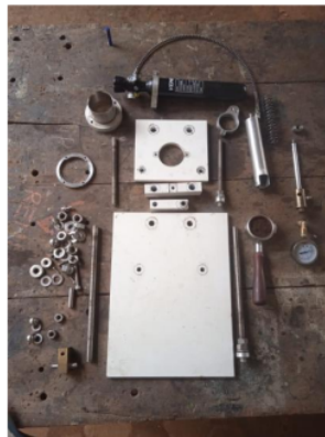
Gambar 4.4 Komponen mesin espresso PCP
