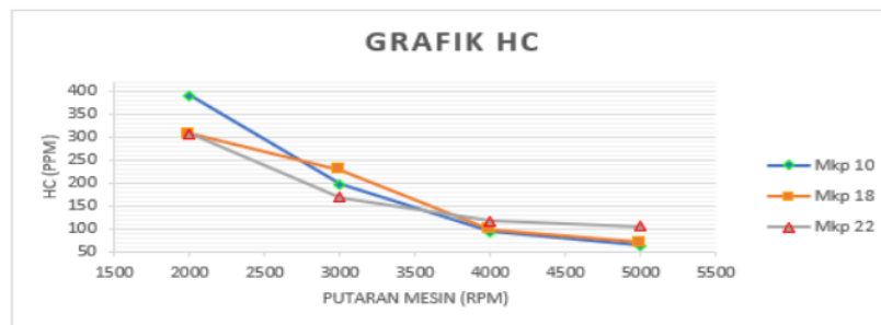
Gambar 2. Hasil Grafik HC
