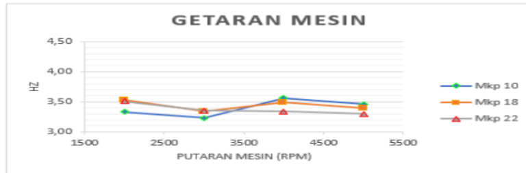
Gambar 4. Hasil Grafik Getaran Mesin
