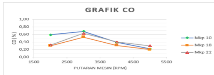
Gambar 3. Hasil Grafik CO
