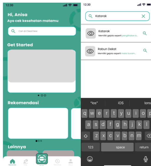
Gambar 6 Tampilan Beranda
