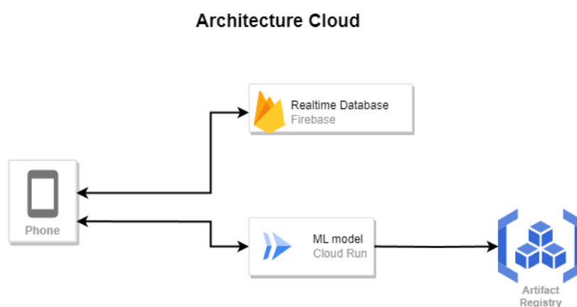
Gambar 1 Arsitektur Cloud
