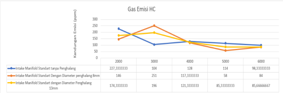
Grafik 4.2 Emisi HC
