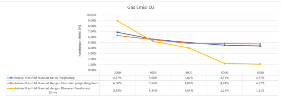
Grafik 4.3 Emisi O 2
