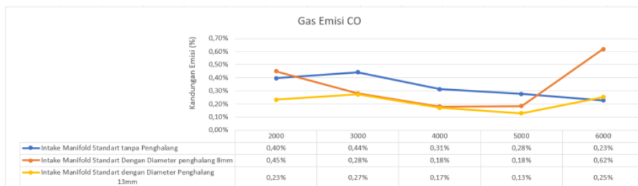
15 Grafik 4.1 Emisi Gas Buang CO
