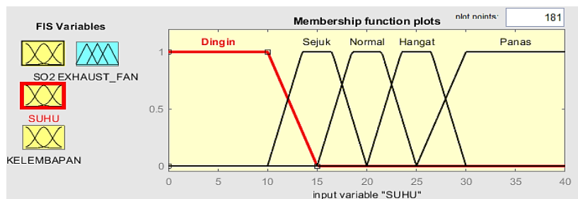
Gambar 3.7 Fungsi Keanggotaan Input Variable Suhu
