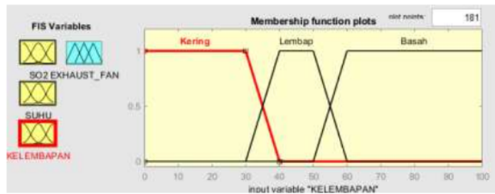
Gambar 3.8 Fungsi Keanggotaan Input Variable Kelembapan
