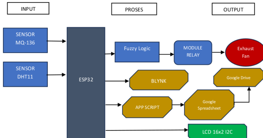
Gambar 3.1 Konsep Blok Sistem
