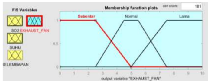
Gambar 3.9 Fungsi Keanggotaan Output Variable Exhaust Fan
