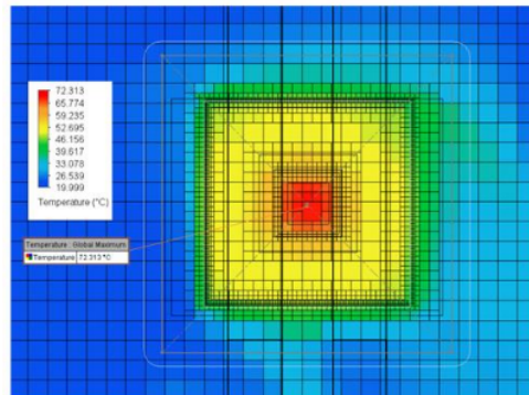
Gambar 4. Hasil Simulasi Pendinginan Hanya dengan Kipas Angin
