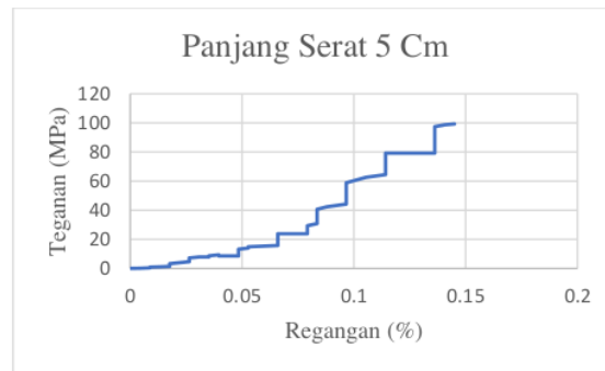
Gambar 6. Tegangan dan Regangan Panjang Serat 5 cm
