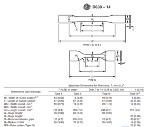
20 Gambar 2. Standar ASTM D638 untuk uji tarik
