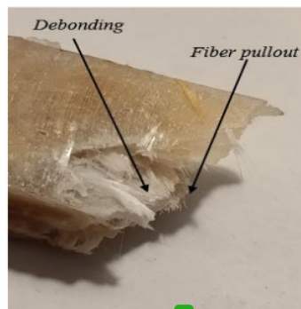
5 Gambar 8. Patahan specimen dengan panjang serat 1 cm
