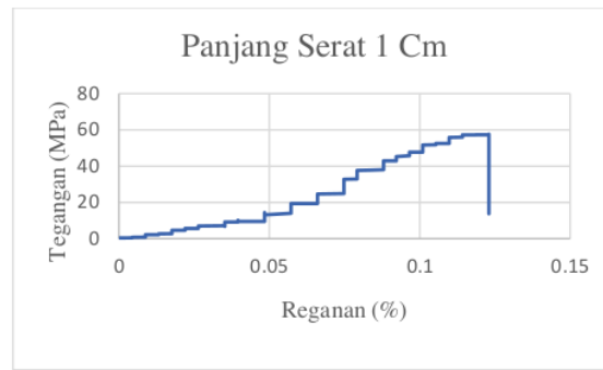
Gambar 4. Tegangan dan Regangan Panjang Serat 1 cm
