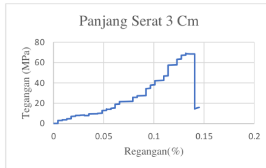
Gambar 5. Tegangan dan Regangan Panjang Serat 3 cm
