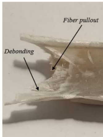
Gambar 10. Patahan specimen dengan panjang serat 5 cm
