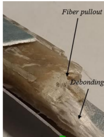
Gambar 9. Patahan specimen dengan panjang serat 3 cm
