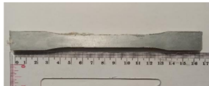
Gambar 1. Spesimen uji tarik komposit FML
