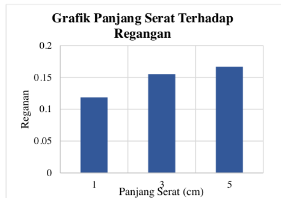
Gambar 7. Regangan terhadap panjang serat
