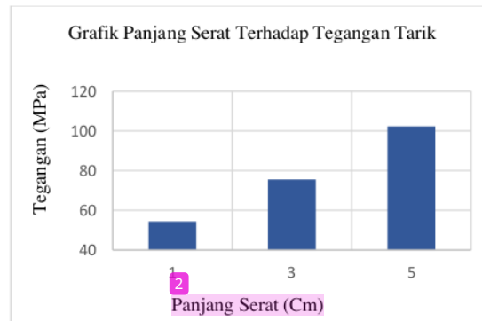
Gambar 3. Diagram panjang serat terhadap tegangan tarik
