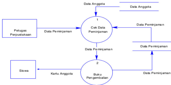
Gambar 8 DFD Level 1 ( proses input data pengembalian )
