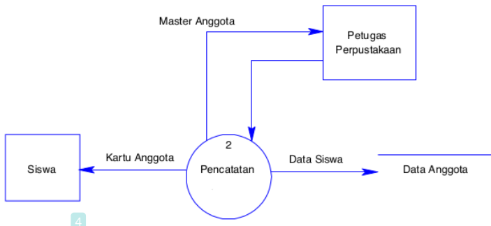
Gambar 5 DFD Level 1 ( proses input data anggota)
