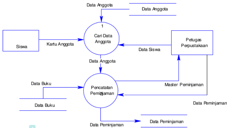
4 Gambar 7 DFD Level 1 ( proses input data peminjam )
