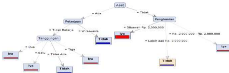
Gambar 18. Hasil Algoritma C4.5
