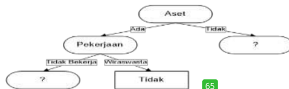
Gambar 4. Pohon Keputusan Node 1.1
