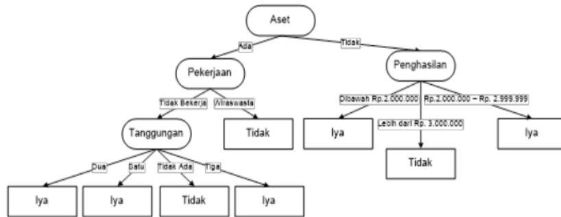
Gambar 6. Pohon Keputusan Node 1.2
