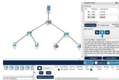
Gambar 7. Pengetesan menggunakan sendmessage
