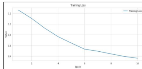
Gambar 3a. Training Loss dengan 3 layer
