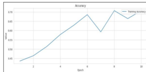
Gambar 1a. Training Accuracy dengan 1 layer
