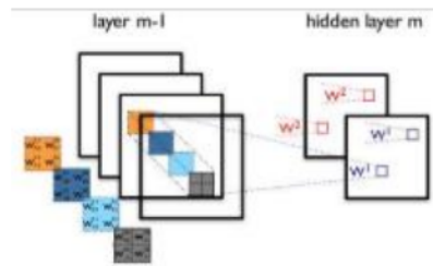
gambar proses Konvolusi pada CNN
