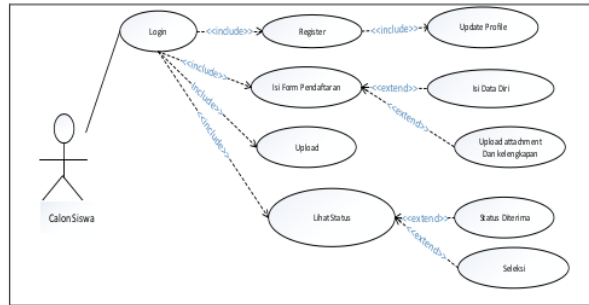
Gambar 3. Use case diagram pendaftaran siswa
