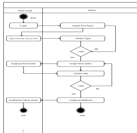
Gambar 9. Activity diagram Siswa melengkapi Form Pendaftaran
