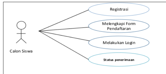
Gambar 2. use case Diagram pendaftaran calon siswa
