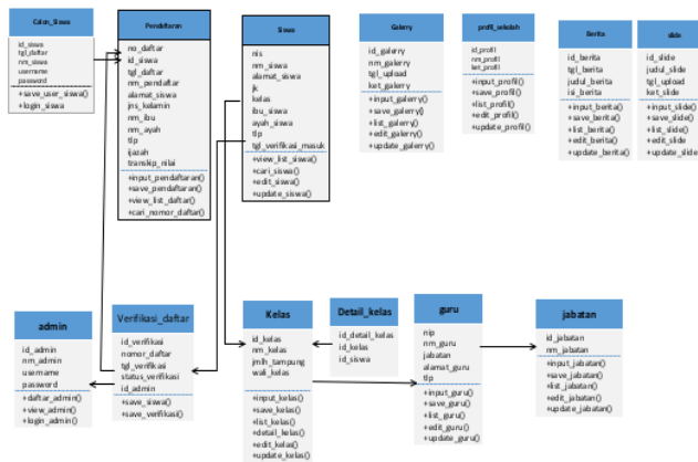
Gambar 7. Class Diagram Pendaftaran siswa baru
