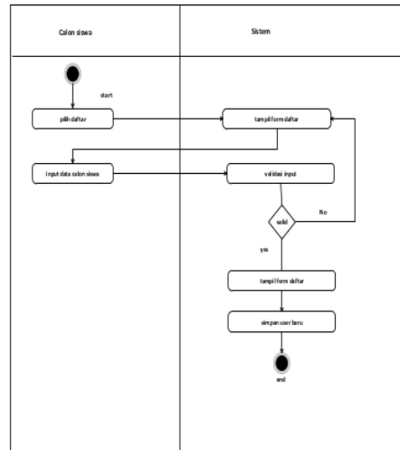
Gambar 8. Activity Diagram Calon Siswa Mendaftarkan Akun Login
