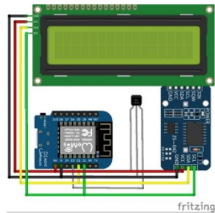
Gambar 3. Skematic
