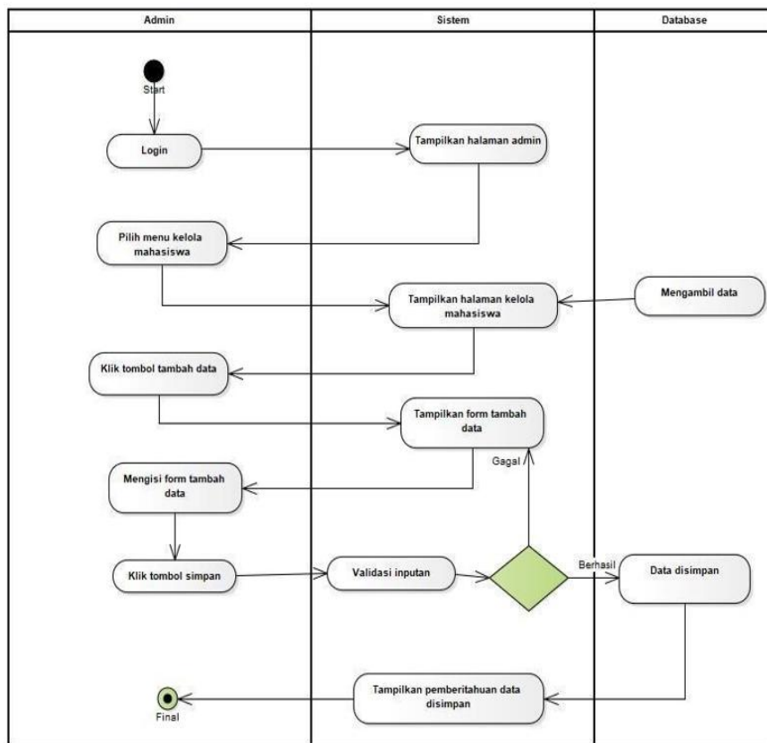
Gambar 3. Activity diagram tambah mahasiswa
