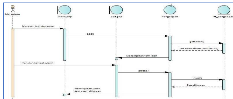
Gambar 5. Sequence diagram unggah dokumen tugas akhir
