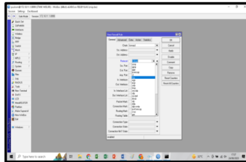
Gambar 3. Pilih Protokol
