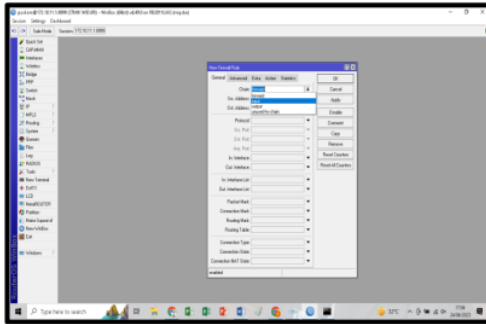
Gambar 2. Membuat Filter
