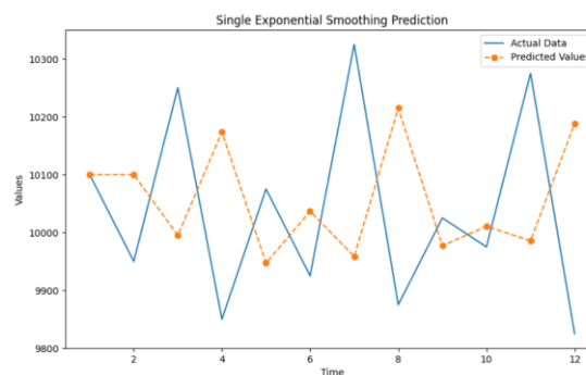
Gambar 4. 55 Grafik SES percobaan 5
