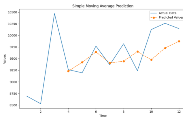
Gambar 4. 40 Grafik SMA percobaan 1
