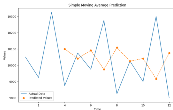
Gambar 4. 52 Grafik SMA percobaan 4
