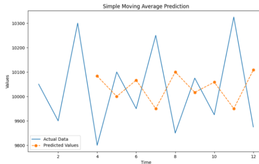
Gambar 4. 44 Grafik SMA percobaan 2
