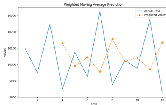
Gambar 4. 57 Grafik WMA percobaan 5
