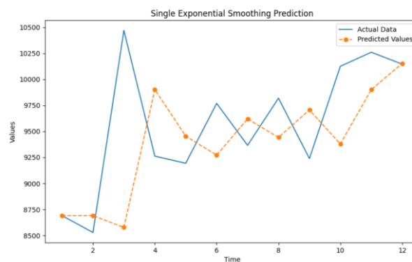
Gambar 4. 39 Grafik SES percobaan 1
