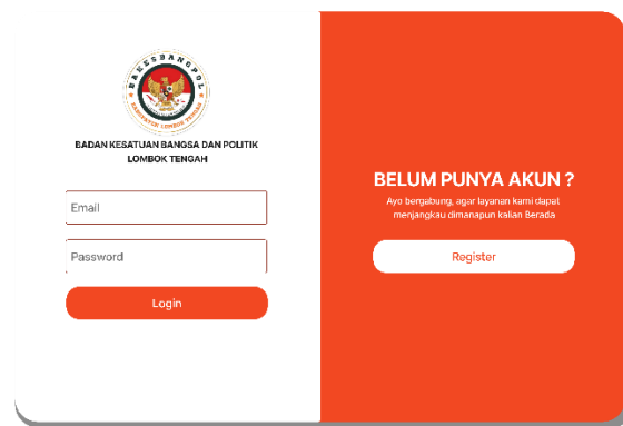
Gambar 4. Halaman Login
