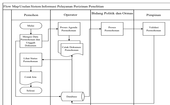
Gambar 2. Sistem Usulan
