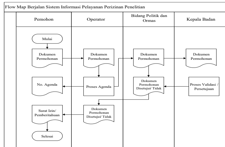
Gambar 1. Sistem Berjalan
