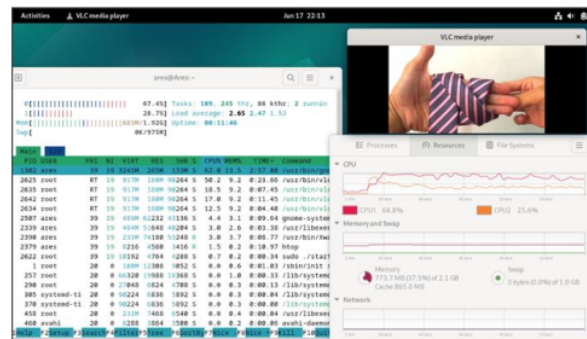
Gambar 4.2.2 Pengujian VLC pada Kernel Real-Time
