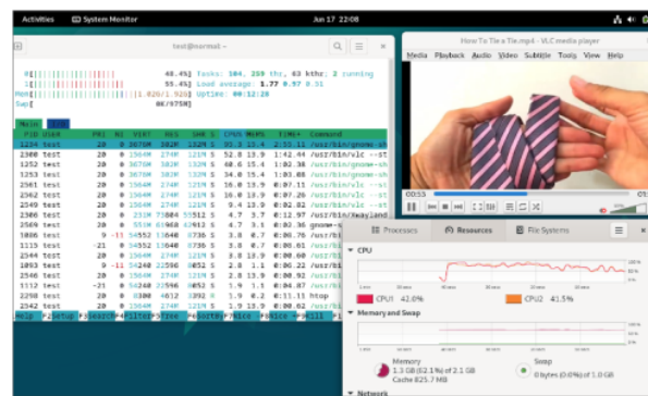
Gambar 4.2.3 Pengujian VLC pada Kernel Normal
