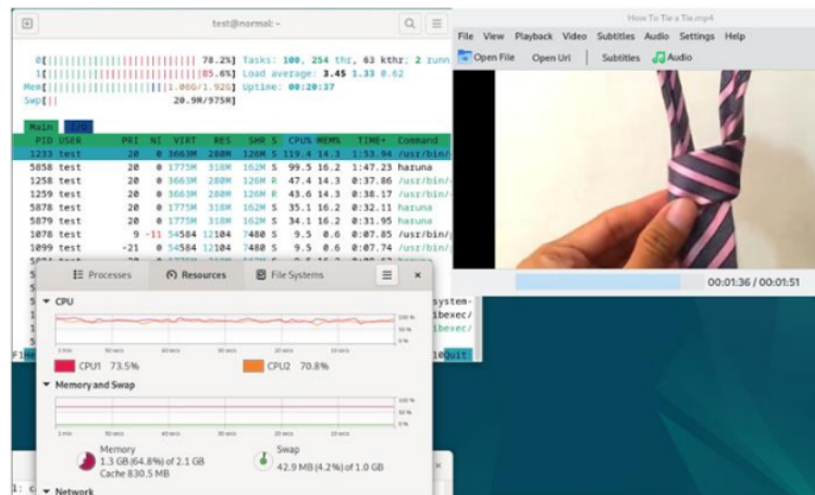
Gambar 4.2.5 Pengujian VLC pada Kernel Normal
