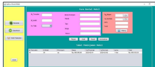
Gambar 6. Halaman Transaksi
