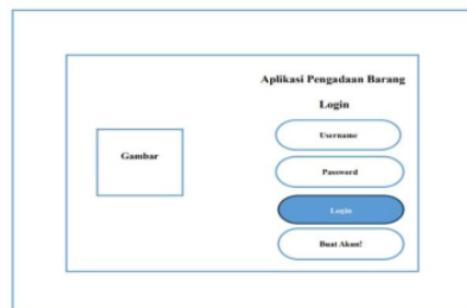
Gambar 5. Halaman Login
