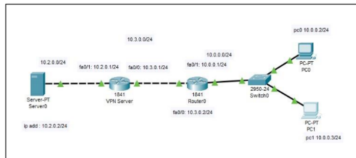
Gambar 1. Simulasi Jaringan
