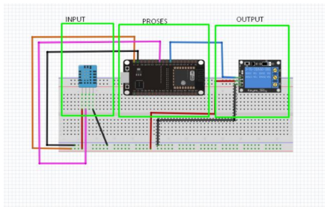
Gambar 3 : Schematic rangkaian alat.
