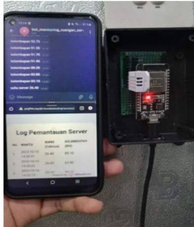
Gambar 5 : Alat mendeteksi suhu dan mengirim notifikasi melalui bot telegram
