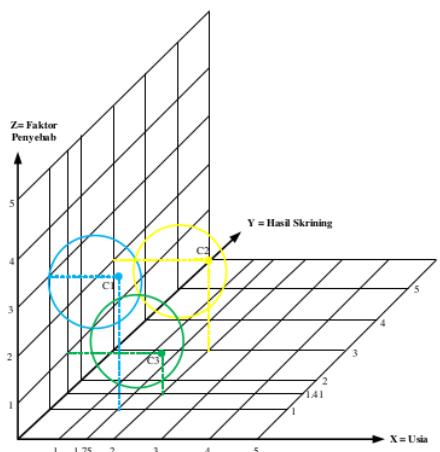
Gambar 4. Grafik Cluster
