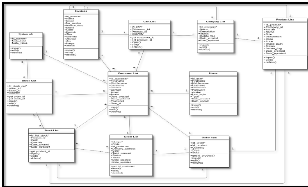
Gambar 4. Class Diagram Sistem Informasi
