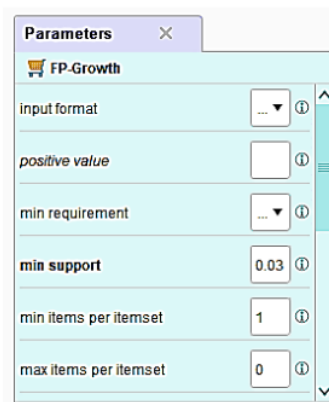
Gambar 6. Tampilan Parameter FP-Growth
