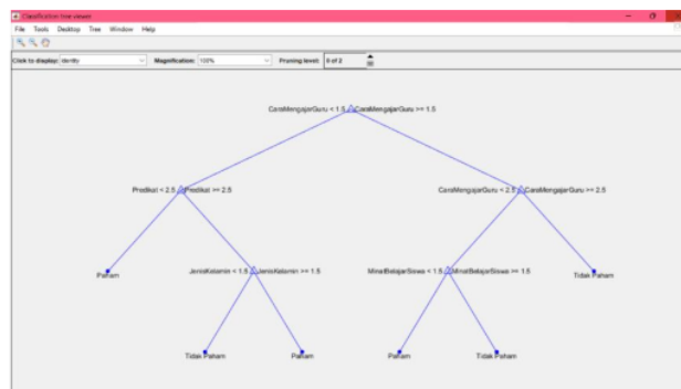
Gambar 4. Hasil Decision Tree C4.5 menggunakan software Matlab
