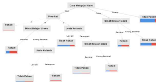
Gambar 1. Hasil Decision Tree C4.5 menggunakan software RapidMiner
