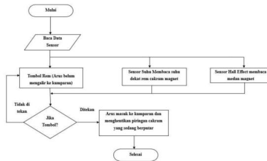
Gambar 2.8 Flowchart dari cara kerja rem magnetik
