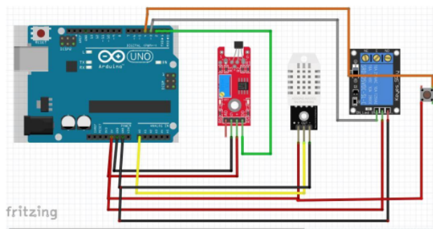
Gambar 2.8 Skematik komponen
