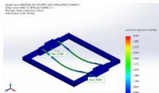
Gambar 5. Pengujian Sumbu X
