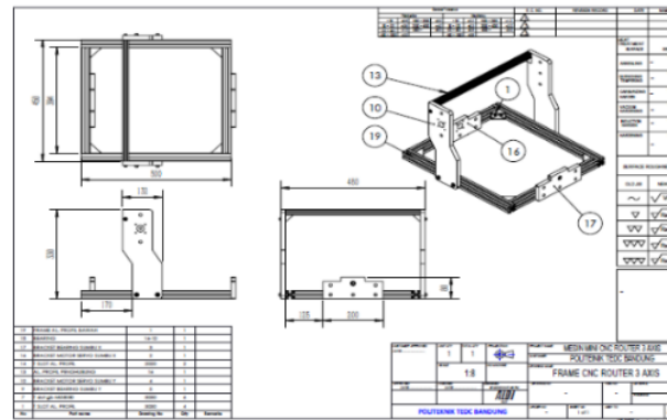
Gambar 4. Desain 2D Bagian Rangka
