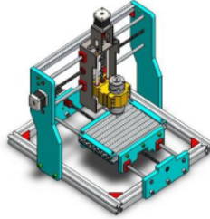
Gambar 2. Desain Mesin CNC Router Mini 3 Axis
