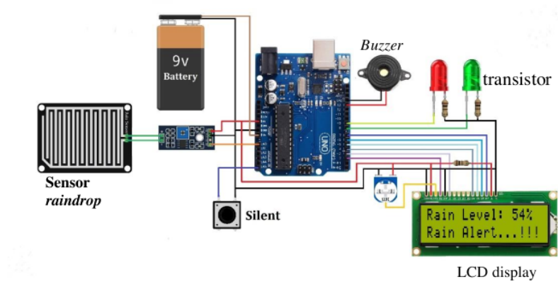
Gambar 3. Perancangan Alat
