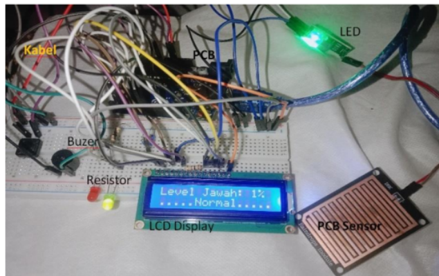
Gambar 4. Rangkaian Detektor Hujan
