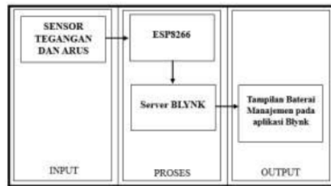
Gambar 3.2 Blok Diagram
