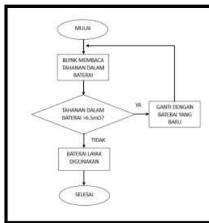
Gambar 3. 3 Flowchart kelayakan baterai
