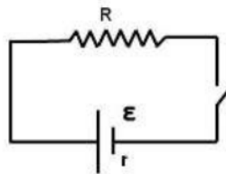
Gambar 2. 4 Rangkaian Rumus Tahanan Dalam
