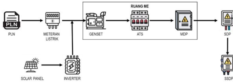
Gambar 26 Konsep Analisis Sistem Elektrikal
