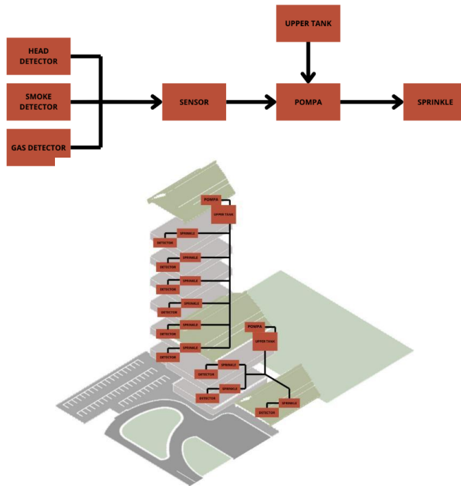
Gambar 27 Sistem Sprinkle
