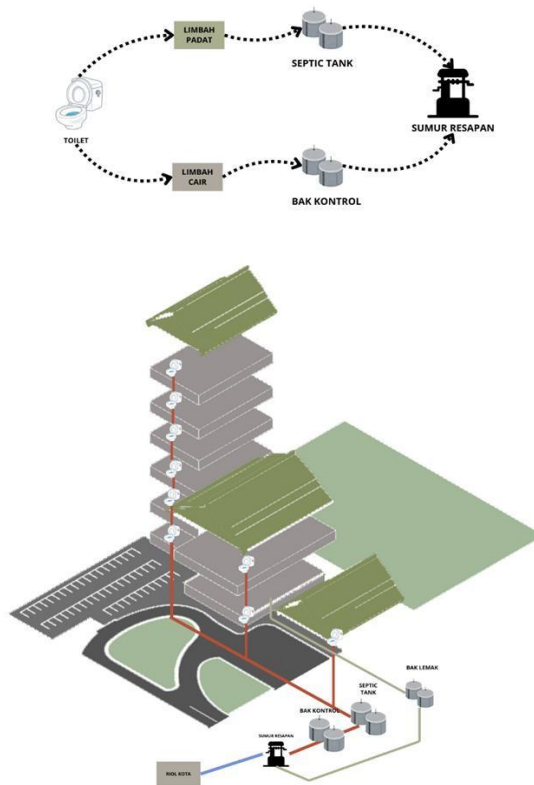
Gambar 24 Konsep Analisis Air Kotor
